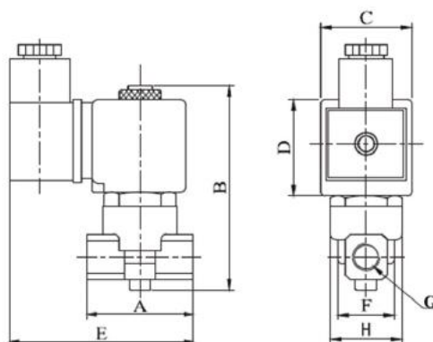
Рис. 5.2 Габаритные и присоединительные размеры клапана типа EV210R
