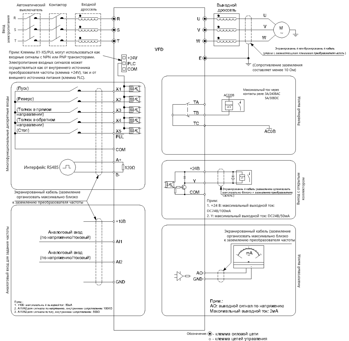
Рисунок 3.5-1 Схема внешних подключений
