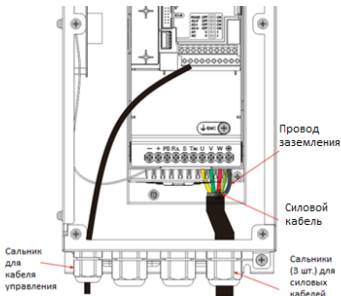
Рисунок 3.4-2 Расположение клемм
