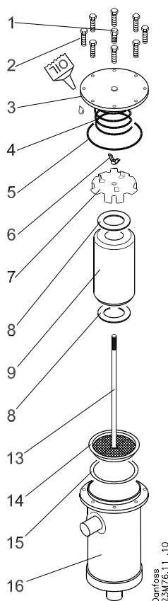
Фильтр DCR с держателем сердечника (один сердечник)
