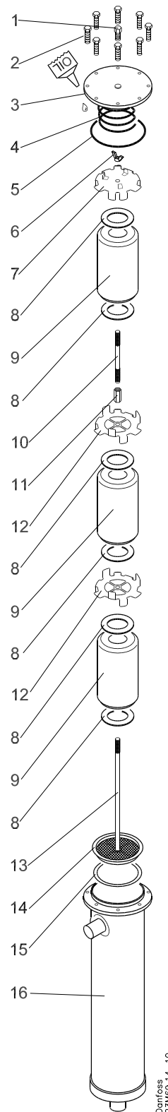
Фильтр DCR с держателем сердечника (три сердечника)
