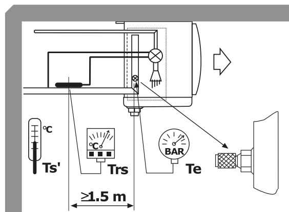
Fig. 5 VERIFICHE CONTROLES COOLER CAPACITY CHECKS LEISTUNGSÜBERPRÜFUNG CONTROLES / КОНТРОЛЬ
